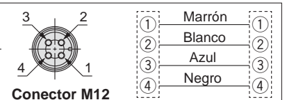
Diagrama de cableado
